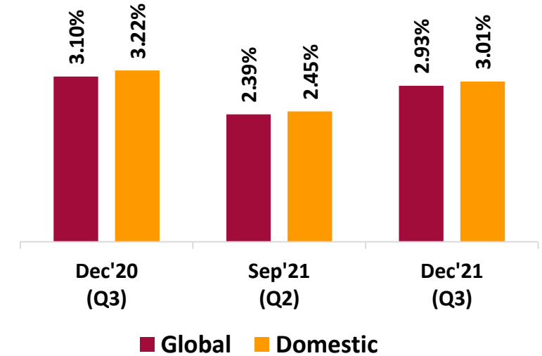
NIM [%]
